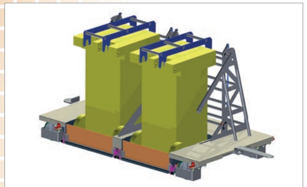
Materialtonnenhalterung mit Routenzug
